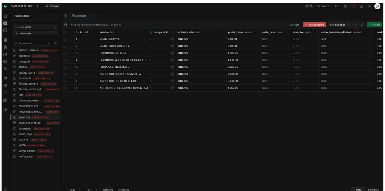
Figura 8. Supabase Studio: las 20 tablas del modelo de datos desplegadas desde database/migraciones/002_modelo_completo.sql, y la tabla producto con registros de prueba.
