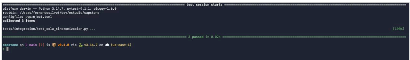
Figura 7. Pruebas de integración de la cola de sincronización, incluido el corte a mitad de sincronización: 3 de 3 en verde (ADR 0002).
